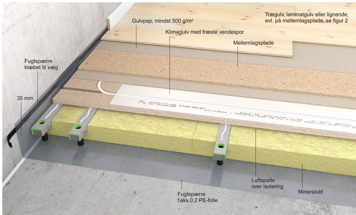
Figur 1 22 eller 25 mm Novopan Klimagulv med fræste vendespor udført efter lægning af gulvpladerne. Vendespor skal udstødtes af en ekstra stålstrø 200 mm fra væg.
