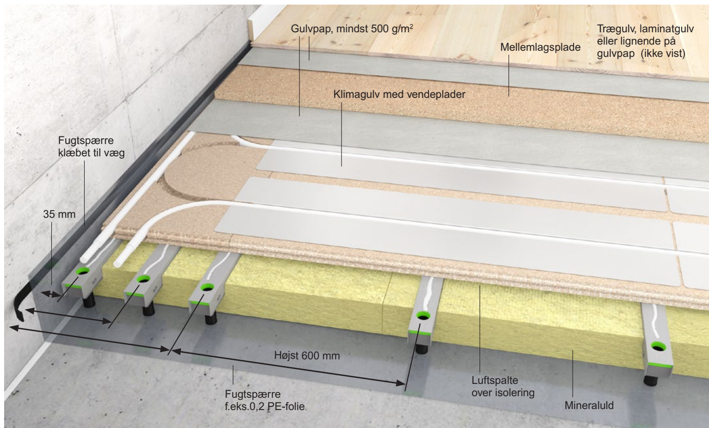
Figur 2 22 eller 25 mm Novopan Klimagulv med vendeplader lagt på stålstrø lang væg og ekstra stålstrøer under vendespor og under samling mellem vendeplader og gulvplader. Mellemlagsplader limes i fer- og notsamlinger og skrues til Klimagulvet, se Faktablad #17 .
